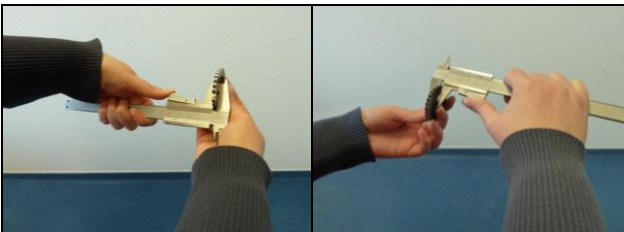
Bild 1/2: Rechtshänder-Schieblehre: Handhabung bei Linkshänder bzw. Rechtshändigkeit (Fotos: C. Kohlhöfer, BGHM)
